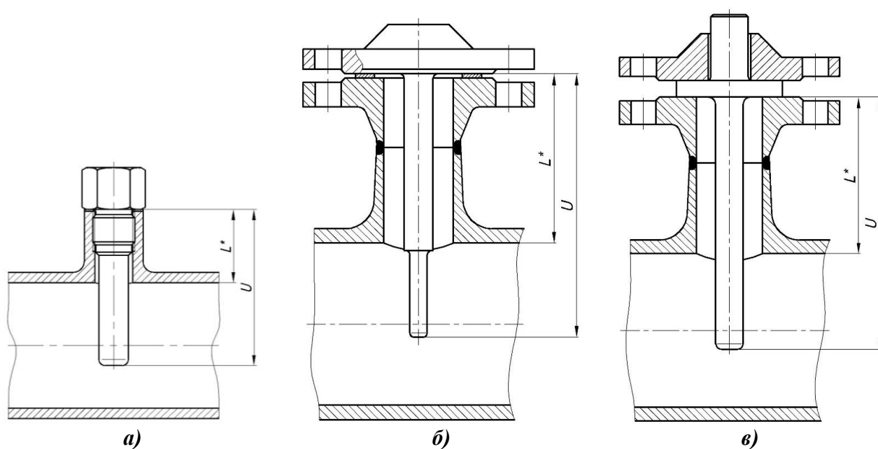
Рис. 7 — Примеры установки гильз защитных на трубопровод
