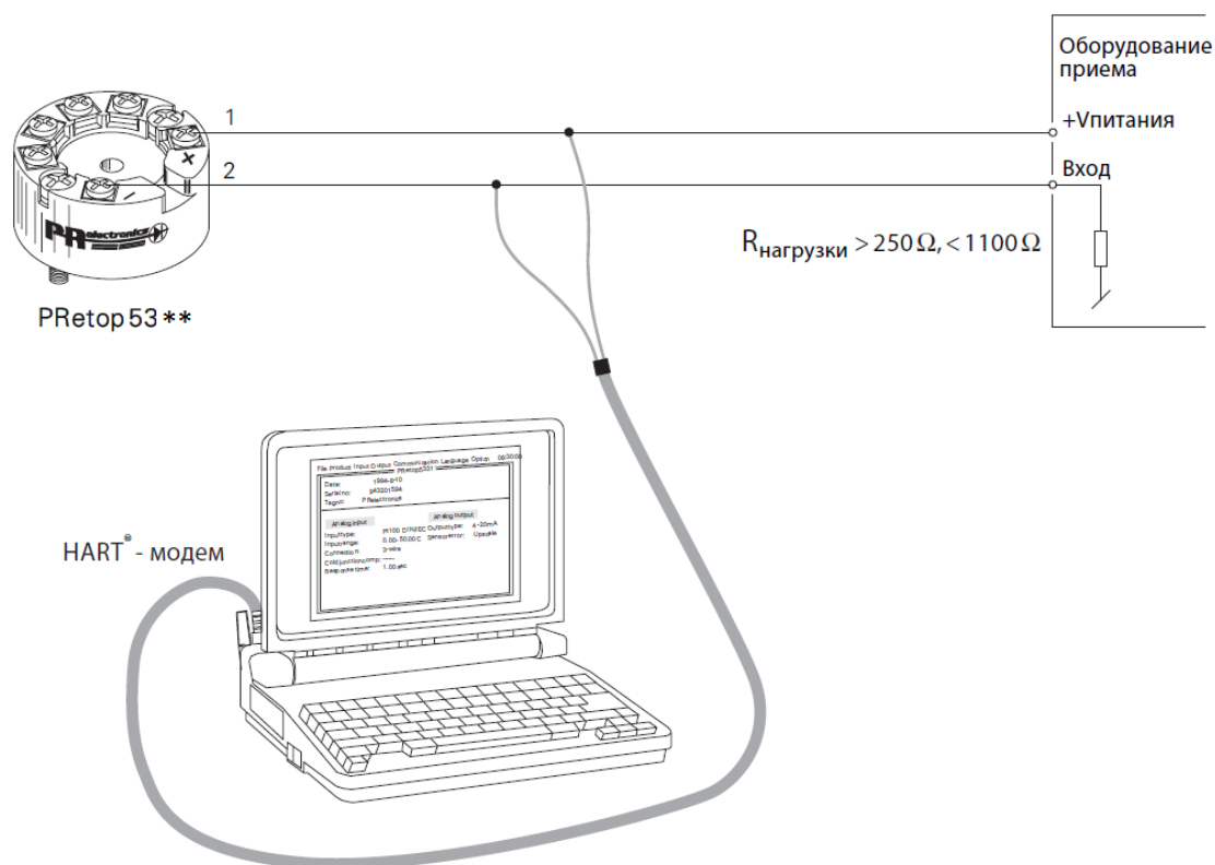
Рис. К.2 — Схема соединений с использованием HART-модема
