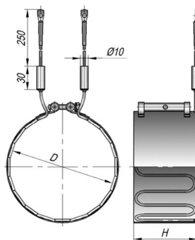
ЭНК-В (воротниковый)
